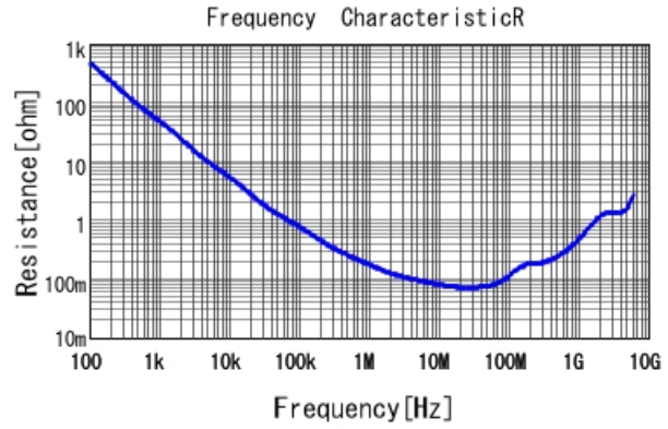
■ GCJ188R71E153KA01 R DC0V, 25degC
