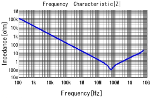
■ GCJ188R71E153KA01 |Z| DC0V, 25degC
