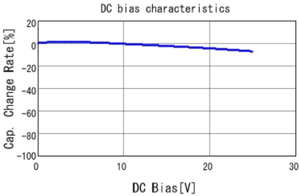
■ GCJ188R71E153KA01 C-DC bias capchange, 25.0degC, AC1.
