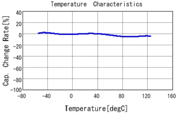
■ GCJ188R71E153KA01 C-Temp. capchange, DCO. 0V, AC1. 0Vrm
