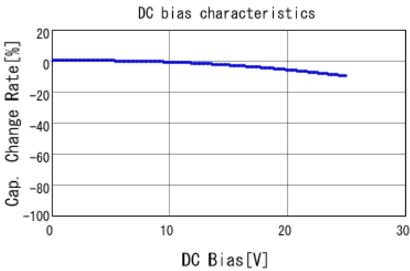
■ GCJ188R71E183KA01 C-DC bias capchange, 25.0degC, AC1.
