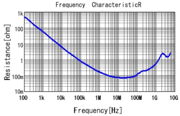
■ GCJ188R71E183KA01 R DC0V, 25degC
