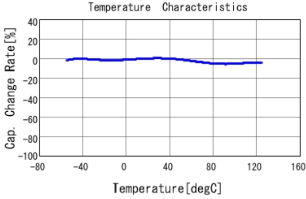
■ GCJ188R71E183KA01 C-Temp. capchange, DCO. 0V, AC1. 0Vrm
