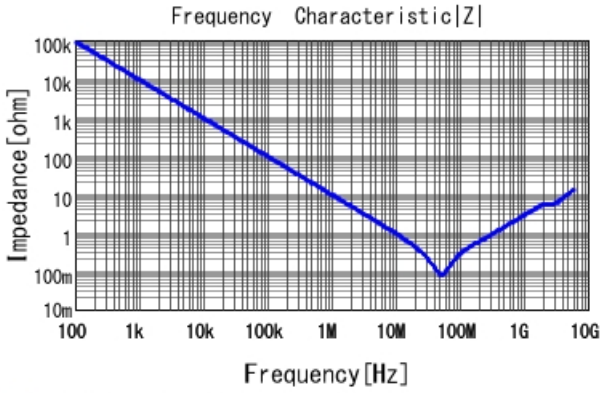
■ GCJ188R71E183KA01 |Z| DC0V, 25degC
