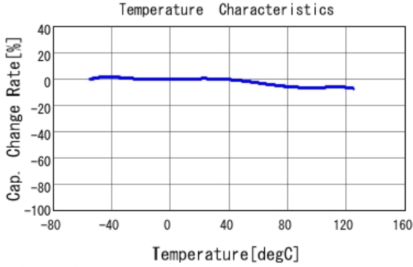
■ GCJ188R71E332KA01 C-Temp. capchange, DCO. 0V, AC1. 0Vrm
