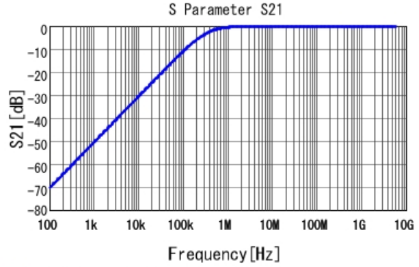
■ GCJ188R71E472KA01 S21 DCOV, 25degC
