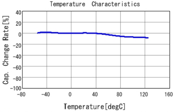
■ GCJ188R71E472KA01 C-Temp. capchange, DCO. 0V, AC1. 0Vrm
