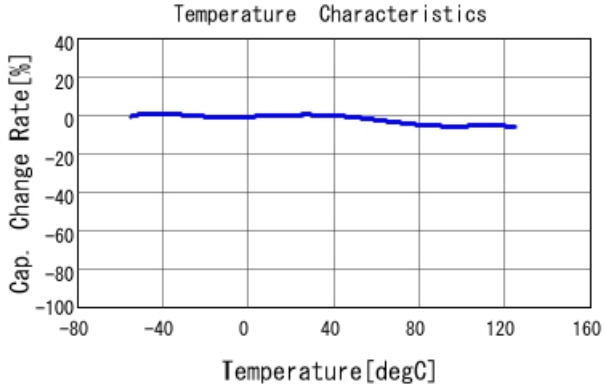
■ GCJ188R71H102KA01 C-Temp. capchange, DCO. 0V, AC1. 0Vrm
