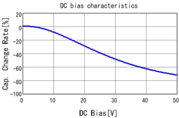
■ GCJ188R71H224KA01 C-DC bias capchange, 25.0degC, AC1.
