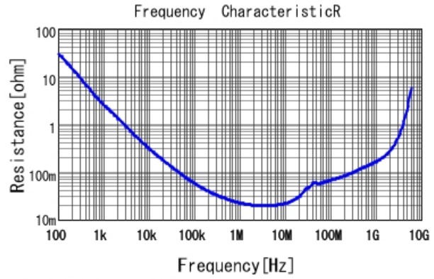
■ GCJ188R71H224KA01 R DC0V, 25degC
