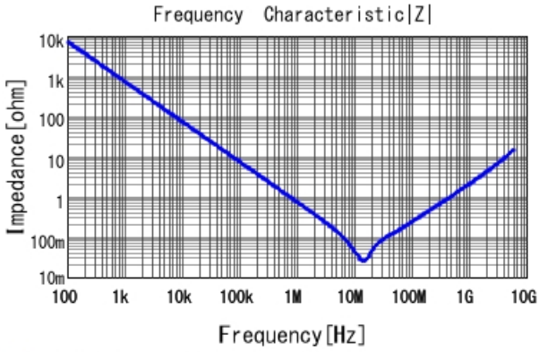
■ GCJ188R71H224KA01 |Z| DC0V, 25degC
