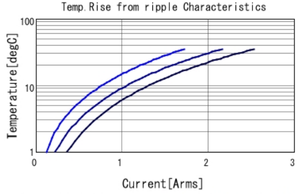
GCJ188R71H224KA01 Temp. rise ■ 300kHz ■ 600kHz ■ 1MHz
