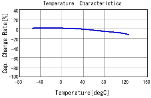
■ GCJ188R71H224KA01 C-Temp. capchange, DCO. 0V, AC1. 0Vrm
