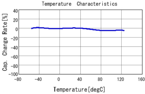
■ GCJ188R71H272KA01 C-Temp. capchange, DCO. 0V, AC1. 0Vrm
