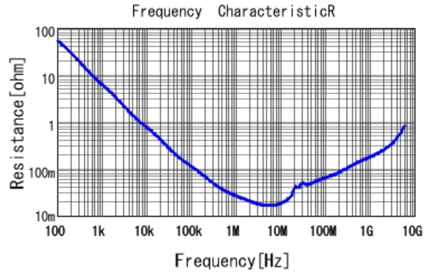
■ GCJ188R91E474KA01 R DC0V, 25degC
