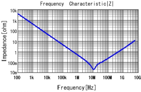
■ GCJ188R91E474KA01 |Z| DC0V, 25degC
