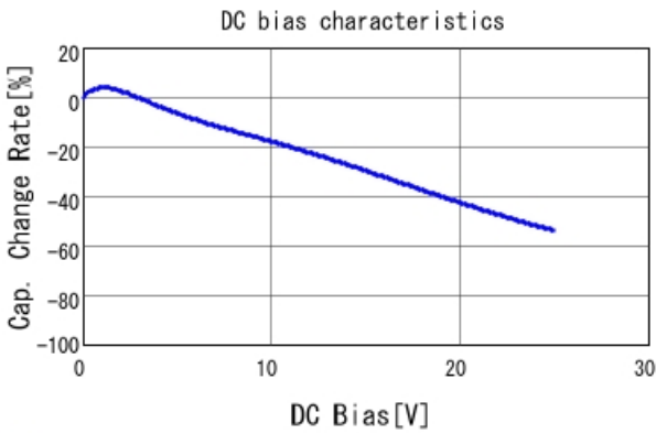
■ GCJ188R91E474KA01 C-DC bias capchange, 25.0degC, AC1.
