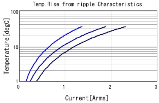
GCJ188R91E474KA01 Temp. rise ■ 200kHz ■ 500kHz ■ 1MHz
