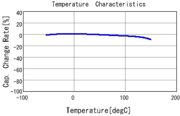
■ GCJ188R91H154KA01 C-Temp. capchange, DCO. 0V, AC1. 0Vrm
