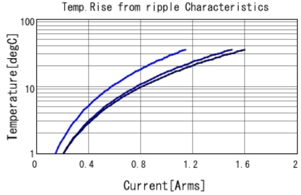
GCJ188R91H154KA01 Temp. rise ■ 400kHz ■ 800kHz ■ 1MHz
