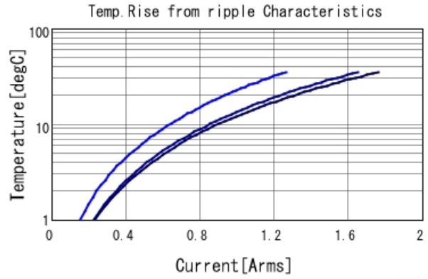
GCJ188R91H184KA01 Temp. rise ■ 400kHz ■ 800kHz ■ 1MHz
