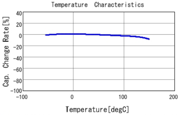
■ GCJ188R91H184KA01 C-Temp. capchange, DCO. 0V, AC1. 0Vrm
