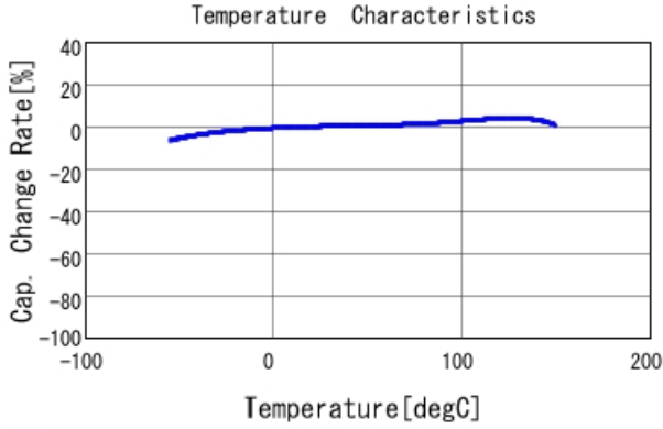
■ GCJ188R92A392KA01 C-Temp. capchange, DCO. 0V, AC1. 0Vrm
