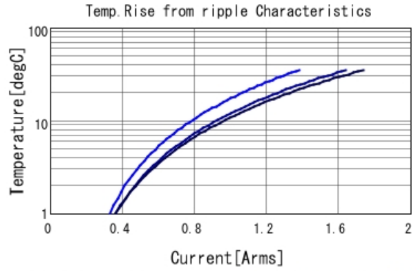
GCJ21BL81E224KA01 Temp. rise ■ 300kHz ■ 600kHz ■ 1MHz
