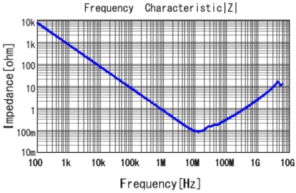
■ GCJ21BL81E224KA01 |Z| DC0V, 25degC
