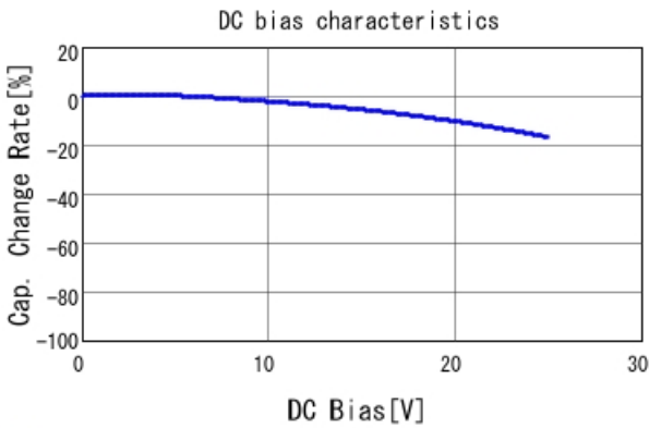
■ GCJ21BL81E224KA01 C-DC bias capchange, 25.0degC, AC1.
