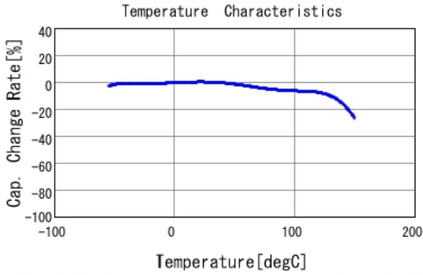
■ GCJ21BL81E224KA01 C-Temp. capchange, DCO. 0V, AC1. 0Vrm
