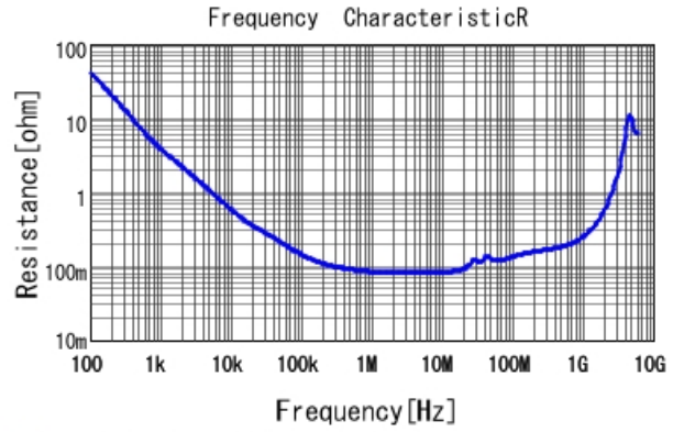
■ GCJ21BL81E224KA01 R DC0V, 25degC
