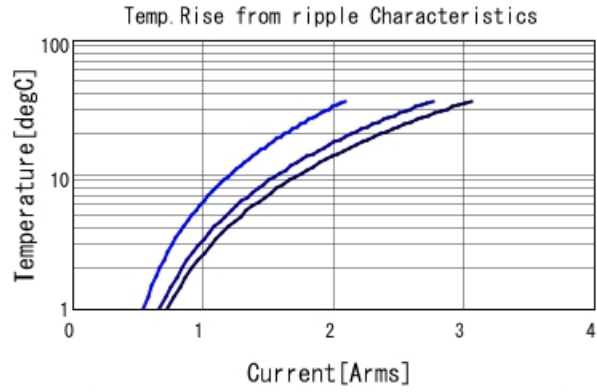
GCJ21BL81E394KA01 Temp. rise ■ 300kHz ■ 600kHz ■ 1MHz
