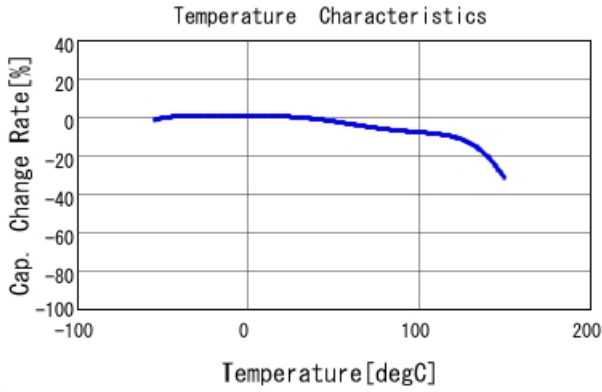
■ GCJ21BL81E394KA01 C-Temp. capchange, DCO. 0V, AC1. 0Vrm
