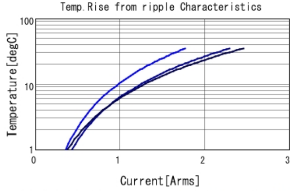
GCJ21BL8YA334KA01 Temp. rise ■ 300kHz ■ 600kHz ■ 1MHz
