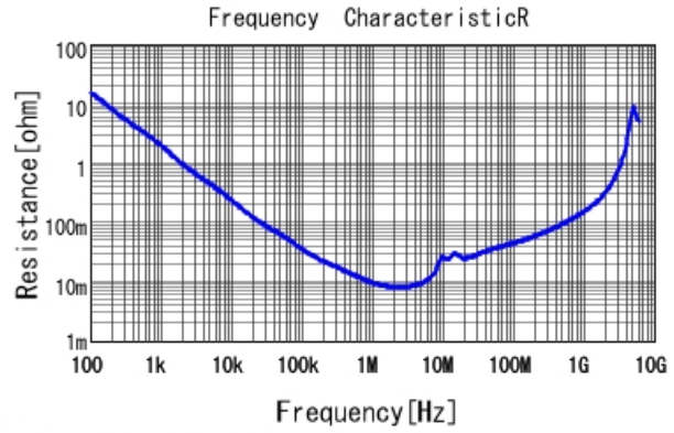
■ GCJ21BR71E225KA01 R DC0V, 25degC
