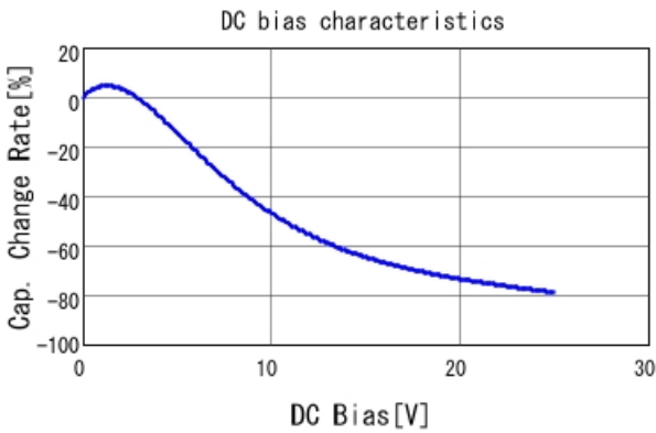
■ GCJ21BR71E225KA01 C-DC bias capchange, 25.0degC, AC1.
