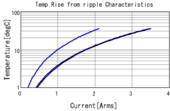
GCJ21BR71E225KA01 Temp. rise ■ 100kHz ■ 500kHz ■ 1MHz
