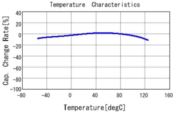
■ GCJ21BR71E225KA01 C-Temp. capchange, DCO. 0V, AC1. 0Vrm
