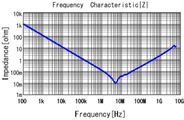
■ GCJ21BR71E225KA01 |Z| DC0V, 25degC
