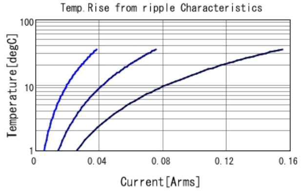
GCJ31BR72J152KXJ1 Temp. rise ■ 30kHz ■ 100kHz ■ 300kHz
