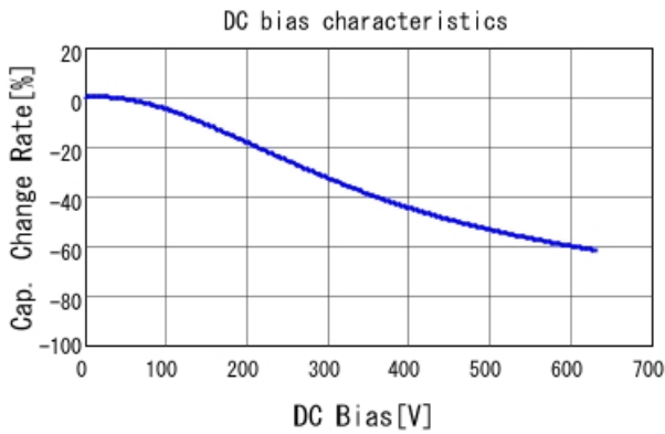
■ GCJ31BR72J152KXJ1 C-DC bias capchange, 25.0degC, AC1V
