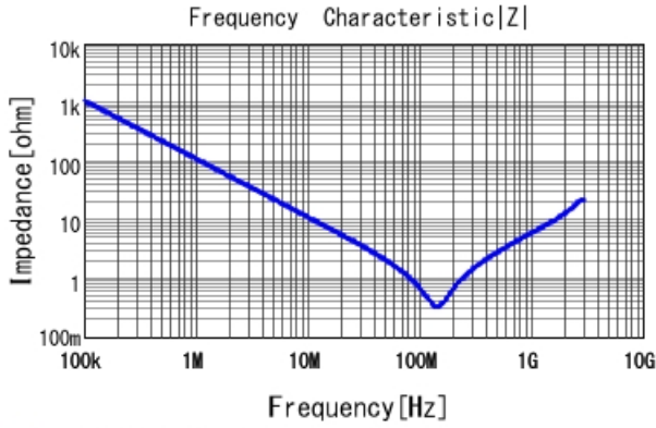
■ GCJ31BR72J152KXJ1 |Z| DC0V, 25degC
