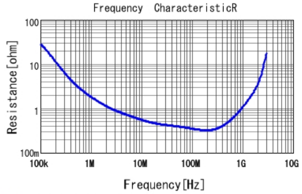
■ GCJ31BR72J152KXJ1 R DC0V, 25degC
