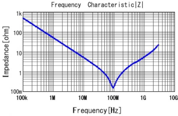
■ GCJ31BR72J332KXJ1 |Z| DC0V, 25degC
