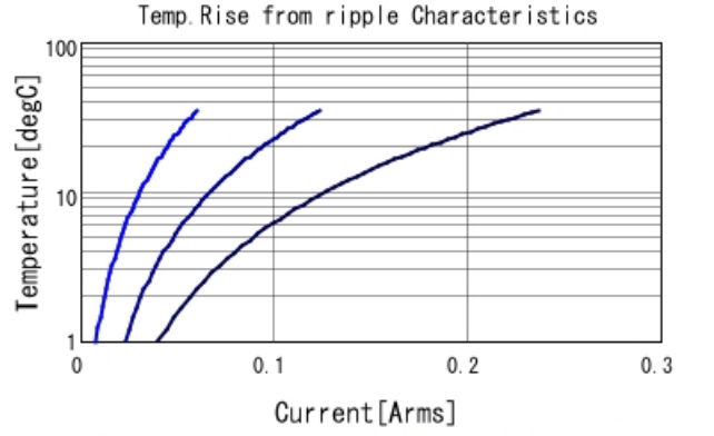
GCJ31BR72J332KXJ1 Temp. rise ■ 30kHz ■ 100kHz ■ 300kHz
