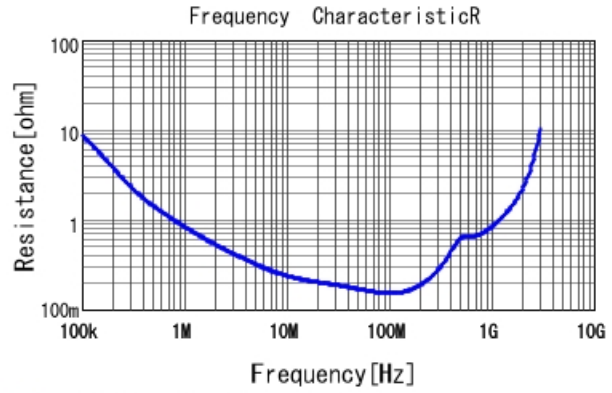
■ GCJ31BR72J332KXJ1 R DC0V, 25degC
