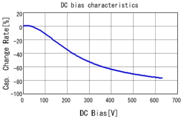
■ GCJ31BR72J332KXJ1 C-DC bias capchange, 25.0degC, AC1V
