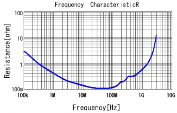
■ GCJ31BR72J682KXJ1 R DC0V, 25degC
