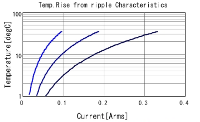
GCJ31BR72J682KXJ1 Temp. rise ■ 30kHz ■ 100kHz ■ 300kHz
