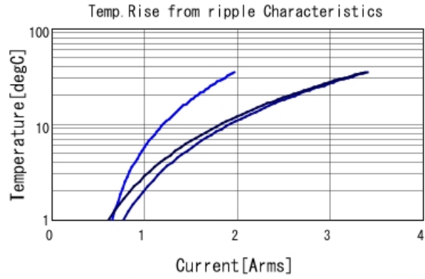
GCJ31CL8YA105KA01 Temp. rise ■ 100kHz ■ 500kHz ■ 1MHz
