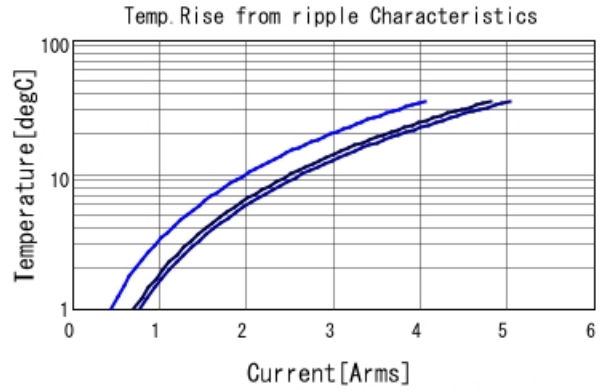
GCJ31CR70J226KE01 Temp. rise ■ 80kHz ■ 400kHz ■ 800kHz
