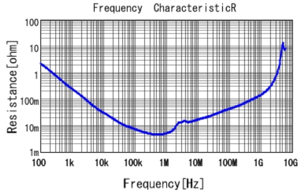
■ GCJ31CR70J226KE01 R DC0V, 25degC
