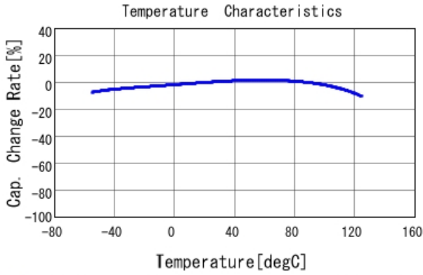
■ GCJ31CR70J226KE01 C-Temp. capchange, DCO. 0V, ACO. 5Vrm
