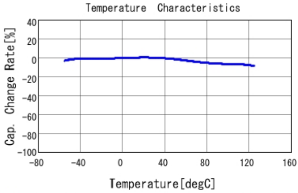
■ GCJ31MR71H474KA01 C-Temp. capchange, DCO. 0V, AC1. 0V rm
