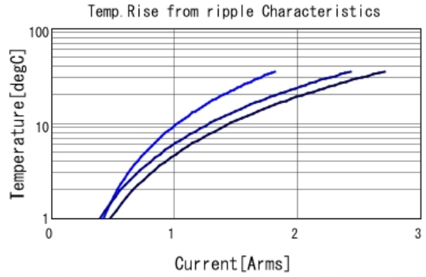
GCJ31MR71H474KA01 Temp. rise ■ 200kHz ■ 500kHz ■ 1MHz
