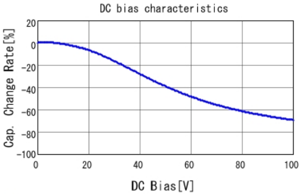
■ GCJ31MR72A184KA01 C-DC bias capchange, 25.0degC, AC1.
