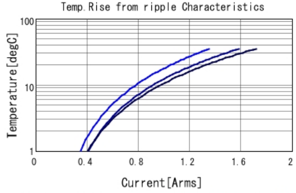
GCJ31MR72A184KA01 Temp. rise ■ 400kHz ■ 800kHz ■ 1MHz
