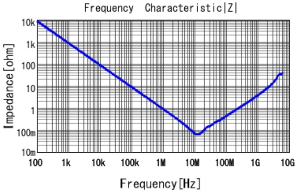
■ GCJ31MR72A184KA01 |Z| DCOV, 25degC
