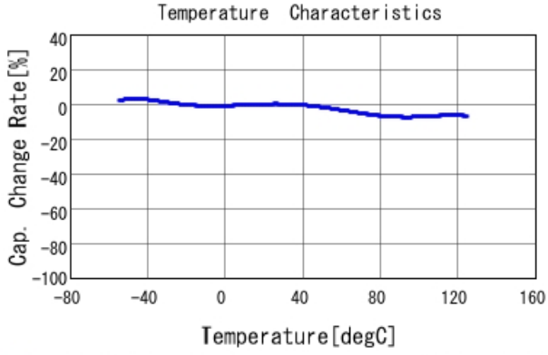
■ GCJ31MR72A184KA01 C-Temp. capchange, DCO. 0V, AC1. 0Vrm
