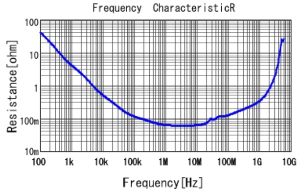
■ GCJ31MR72A184KA01 R DCOV, 25degC
