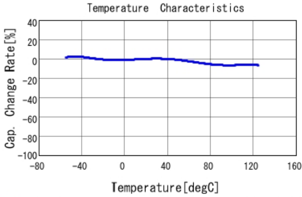
■ GCJ31MR72A224KA01 C-Temp. capchange, DCO. 0V, AC1. 0Vrm
