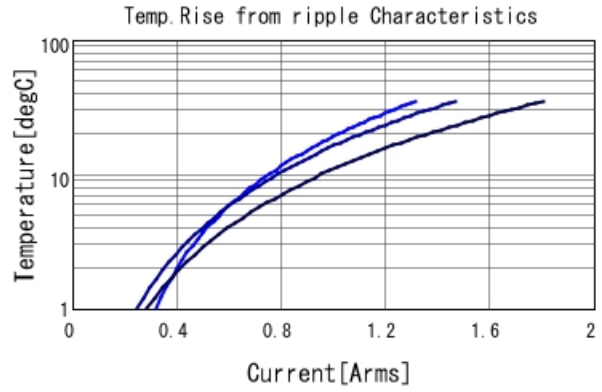
GCJ31MR72A224KA01 Temp. rise ■ 300kHz ■ 600kHz ■ 1MHz
