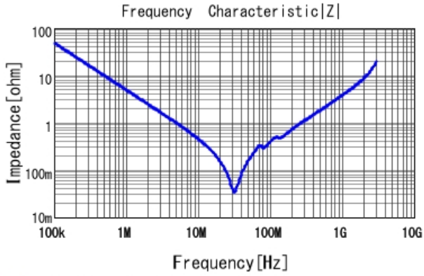
■ GCJ32DR72J333KXJ1 |Z| DC0V, 25degC
