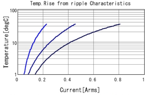
GCJ32DR72J333KXJ1 Temp. rise ■ 30kHz ■ 100kHz ■ 300kHz
