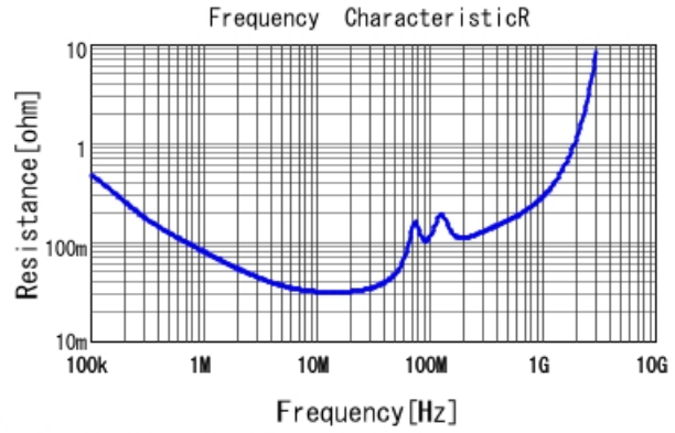
■ GCJ32DR72J333KXJ1 R DC0V, 25degC
