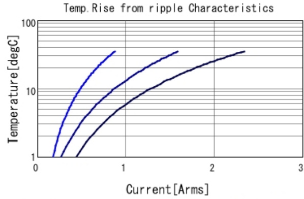
■ GCJ43DR72E474KXJ1 Temp. rise ■ 30kHz ■ 100kHz ■ 300kHz
