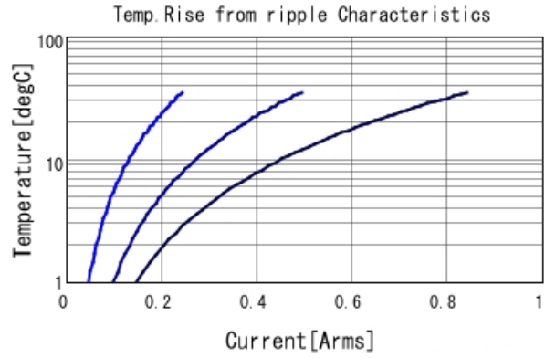
GCJ43DR72J333KXJ1 Temp. rise ■ 30kHz ■ 100kHz ■ 300kHz
