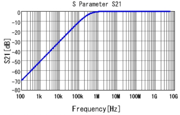
■ GCM155L81H472KA37 S21 DCOV, 25degC
