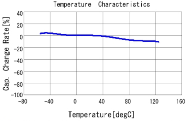
■ GCM155R71E103KA37 C-Temp. capchange, DCO. 0V, AC1. 0Vrm
