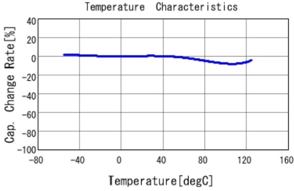
■ GCM155R71H221KA37 C-Temp. capchange, DCO. 0V, AC1. 0Vrm
