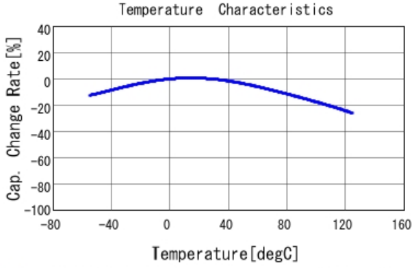
■ GCM188D70G106ME36 C-Temp. capchange, DCO. 0V, ACO. 2Vrm
