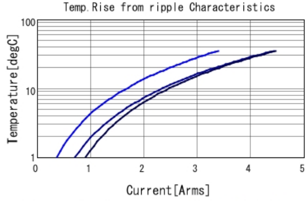
GCM188D70G106ME36 Temp. rise ■ 80kHz ■ 400kHz ■ 800kHz
