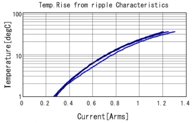
GQM2195G2E470JB12 Temp. rise ■ 500MHz ■ 700MHz ■ 1GHz
