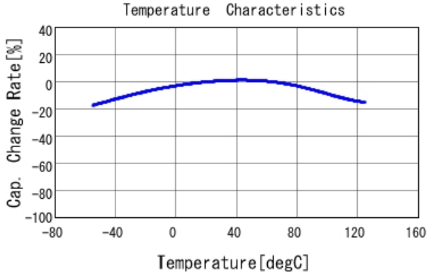
■ GRJ188C70J475KE11 C-Temp. capchange, DCO. 0V, ACO. 2Vrm
