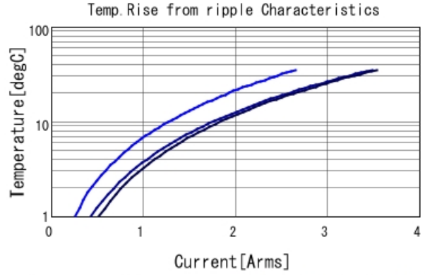
GRJ188C70J475KE11 Temp. rise ■ 100kHz ■ 500kHz ■ 1MHz
