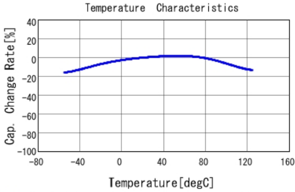
■ GRM033C71C104KE14 C-Temp. capchange, DCO. 0V, ACO. 2Vrm
