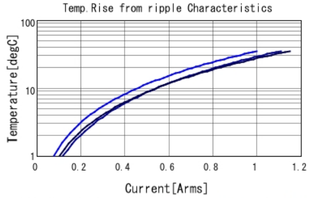
GRM033C71C104KE14 Temp. rise ■ 400kHz ■ 800kHz ■ 1MHz
