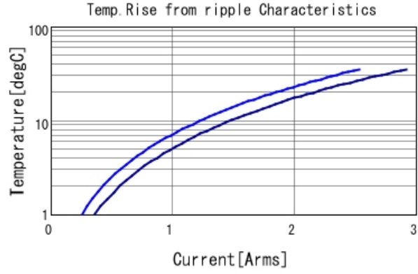
GRM033C80J105ME05 Temp. rise ■ 500kHz ■ 1MHz
