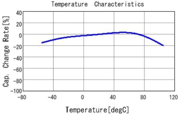
■ GRM033C80J105ME05 C-Temp. capchange, DCO. 0V, ACO. 1Vrm
