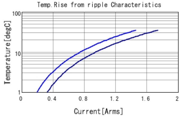
GRM033C80J224KE90 Temp. rise ■ 600kHz ■ 1MHz
