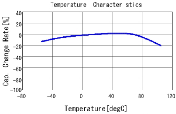
■ GRM033C80J224KE90 C-Temp. capchange, DCO. 0V, ACO. 1Vrm
