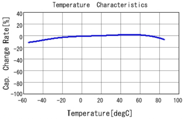
■ GRM033R60G105MEA2 C-Temp. capchange, DCO. 0V, ACO. 1Vrm
