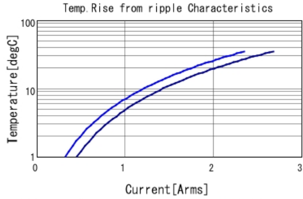
GRM033R60G105MEA2 Temp. rise ■ 500kHz ■ 1MHz
