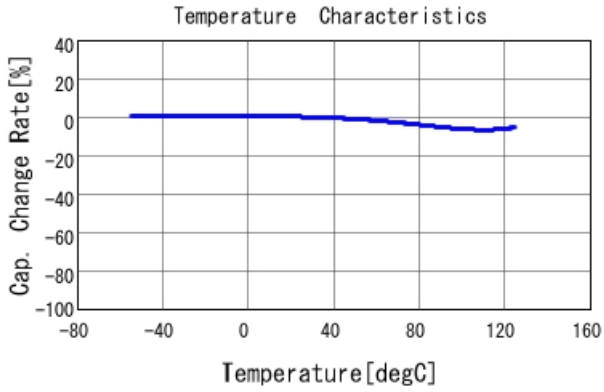
■ GRM033R71E681KA01 C-Temp. capchange, DCO. 0V, AC1. 0Vrm
