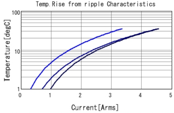
GRM155R60E475ME76 Temp. rise ■ 100kHz ■ 500kHz ■ 1MHz
