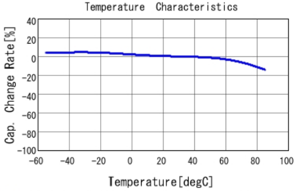
■ GRM155R60E475ME76 C-Temp. capchange, DCO. 0V, ACO. 5Vrm
