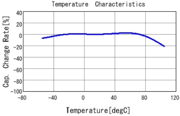
■ GRM21BC81C106KE15 C-Temp. capchange, DCO. 0V, ACO. 5Vrm
