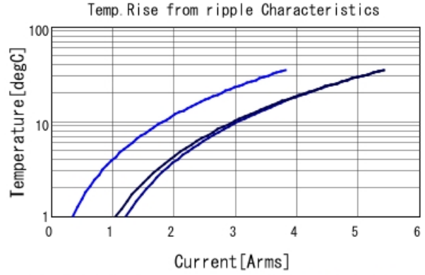
GRM21BC81C106KE15 Temp. rise ■ 80kHz ■ 400kHz ■ 800kHz
