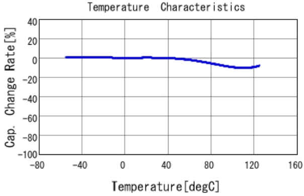
■ GRM21BR72A473KA01 C-Temp. capchange, DCO. 0V, AC1. 0Vrm
