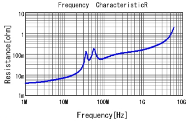
■ GRM3195C1H104JA05 R DCOV, 25degC
