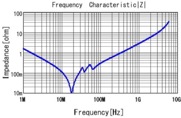
■ GRM3195C1H104JA05 |Z| DCOV, 25degC
