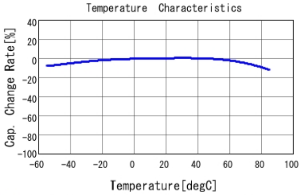
■ GRM319R61C226KE15 C-Temp. capchange, DCO. 0V, ACO. 5Vrm
