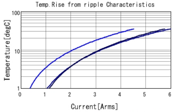
GRM319R61C226KE15 Temp. rise ■ 80kHz ■ 400kHz ■ 800kHz
