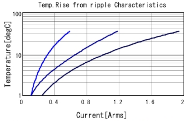
GRM43QR72E154KW01 Temp. rise ■ 30kHz ■ 100kHz ■ 300kHz
