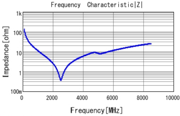
■ GRT1555C1E120JA02 |Z| DC0V, 25degC
