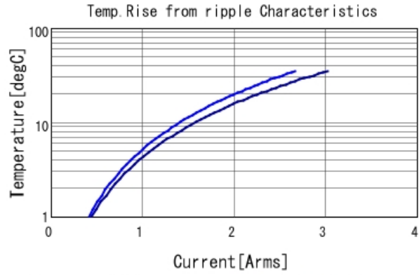
■ GRT155C71A105KE13 Temp. rise ■ 500kHz ■ 1MHz
