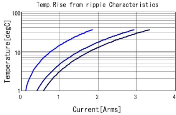
■ GRT155C81C105KE13 Temp. rise ■ 100kHz ■ 500kHz ■ 1MHz
