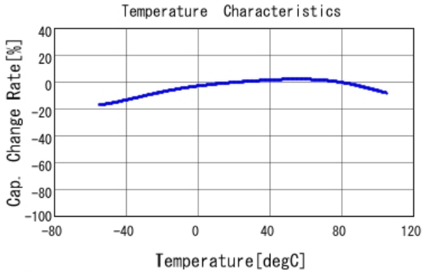
■ GRT155C81C105KE13 C-Temp. capchange, DCO. 0V, ACO. 2V rm
