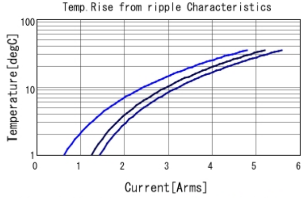
■ GRT188C80G226ME13 Temp. rise ■ 80kHz ■ 400kHz ■ 800kHz
