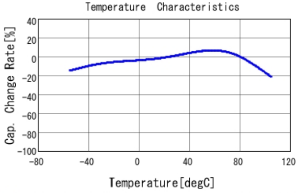
■ GRT188C80G226ME13 C-Temp. capchange, DCO. 0V, ACO. 1Vrm
