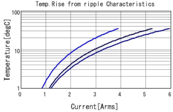
■ GRT32DC81H335KE01 Temp. rise ■ 100kHz ■ 500kHz ■ 1MHz
