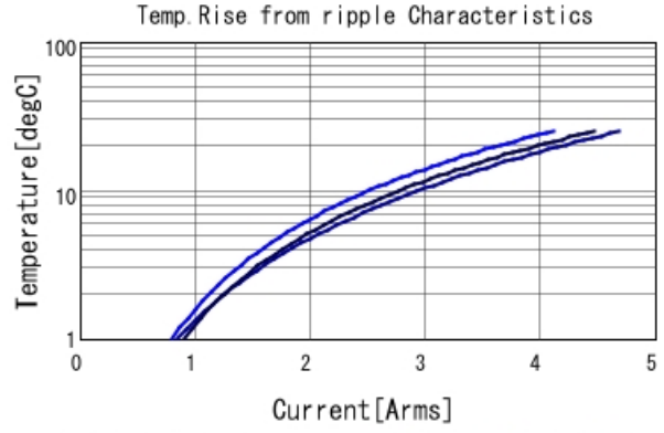
KRM55QR71J106KH01 Temp. rise ■ 50kHz ■ 100kHz ■ 300kHz
