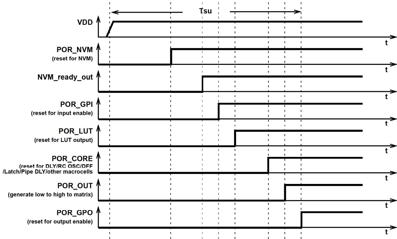
Figure 43. POR sequence
